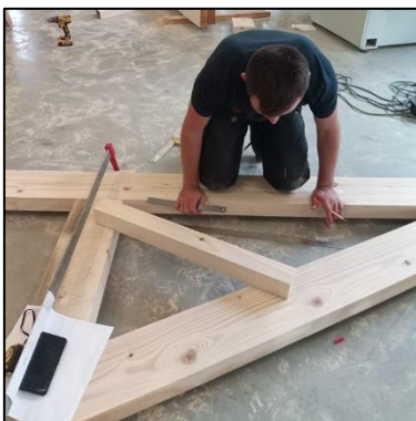
Tracé des contrefiches
